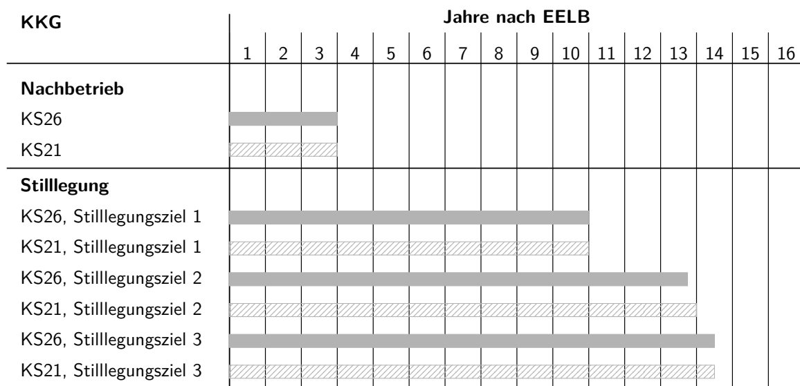
Abbildung 7: Voraussichtliche Dauer der Stilllegungs- und Rückbauarbeiten ab EELB für KKG.
