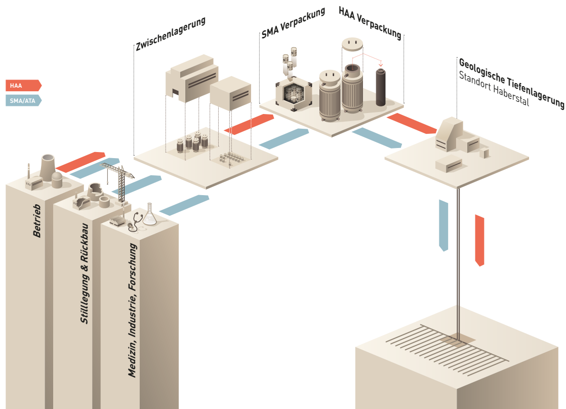
Abbildung 2: Übergeordnete Elemente der Entsorgung in der Schweiz.
