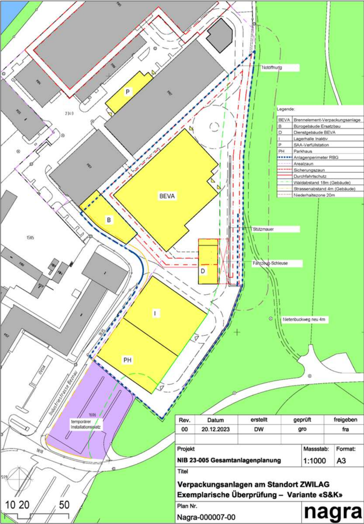
Abbildung 7: Übersichtsplan der modellhaften Anordnung der Oberflächeninfrastruktur am Standort Würenlingen.
