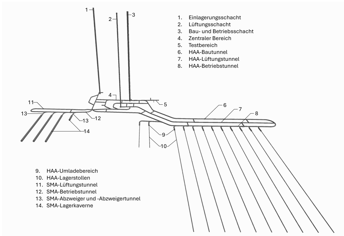
Abbildung 8: Anlagenkonzept der untertägigen Anlagen und Bauten für das KS26-Basisprojekt.
