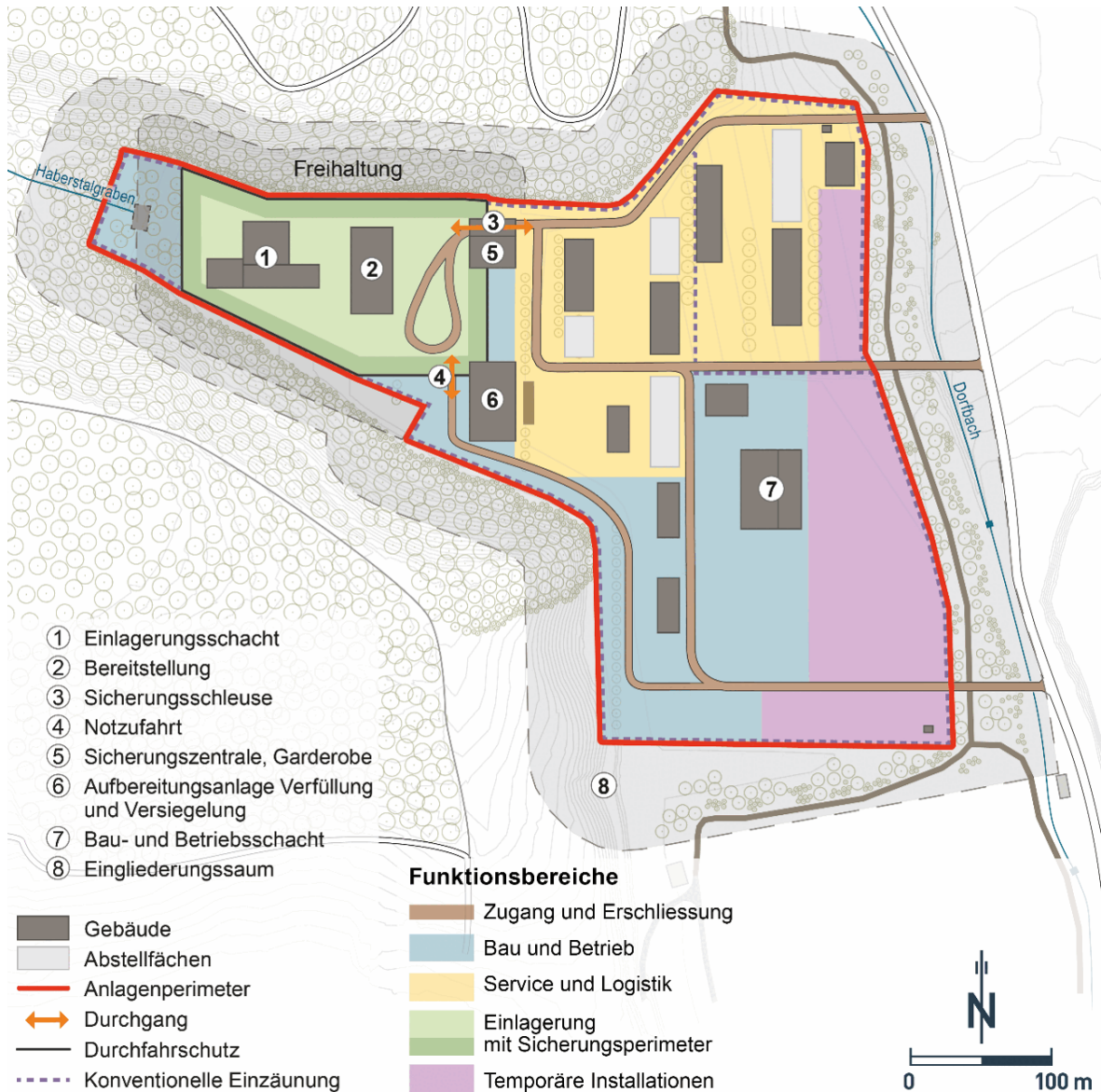
Abbildung 10: Übersichtsplan der modellhaften Anordnung der Oberflächeninfrastruktur der KS26-Perspektive am Standort Haberstal.
