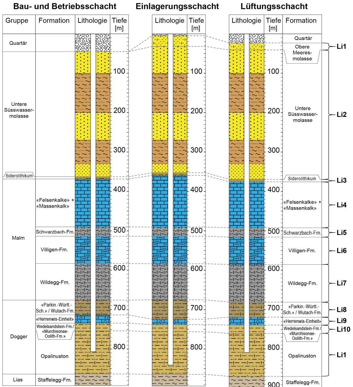
Abbildung 9: Gegenüberstellung der prognostizierten lithologischen Einheiten in den geplanten Zugangsbauwerken des KS26-Basisprojektes [18].
