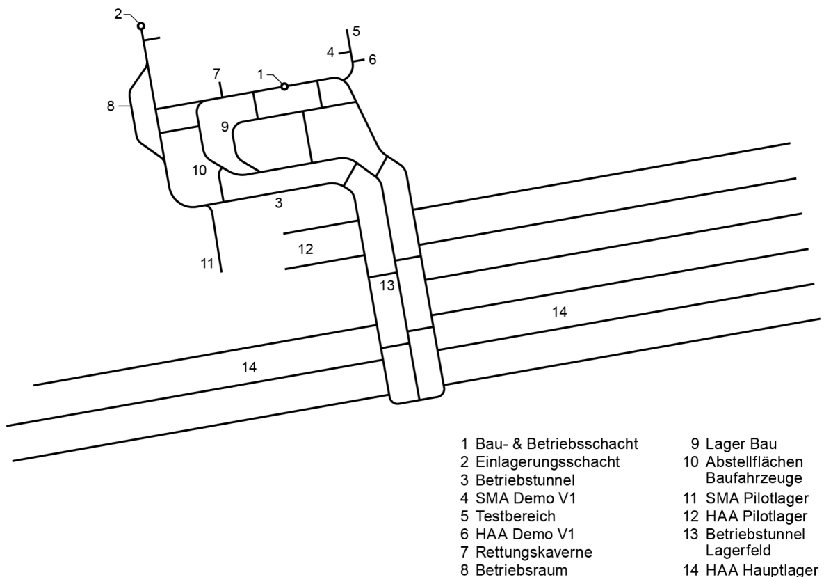
Abbildung 11: Systemskizze für die untertägigen Anlagenelemente und Bauten des Tiefenlagers gemäss KS26-Perspektive.
